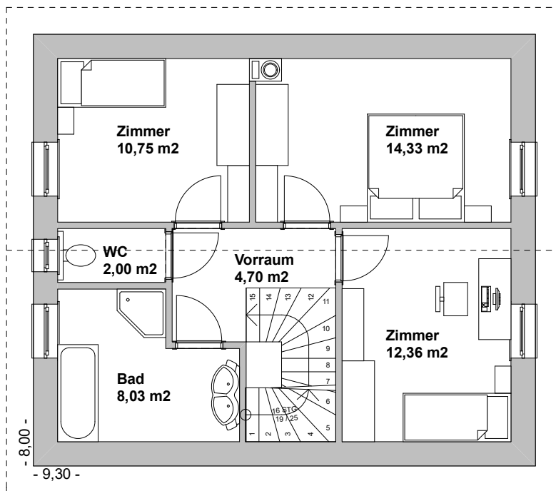
Obergeschoss M 1:100 - WNF = 52,17 m 2
