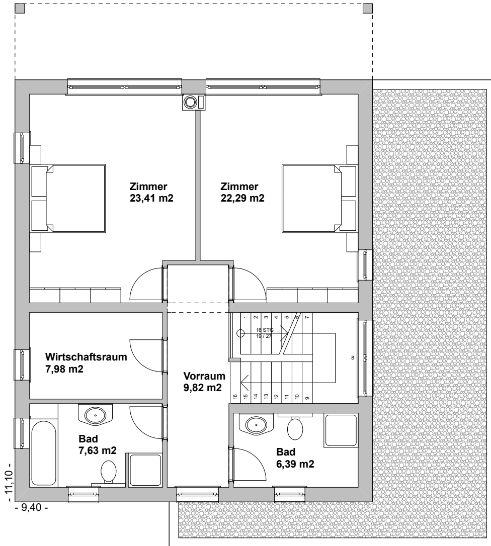
Obergeschoss M 1:100 - WNF = 77,52 m 2
