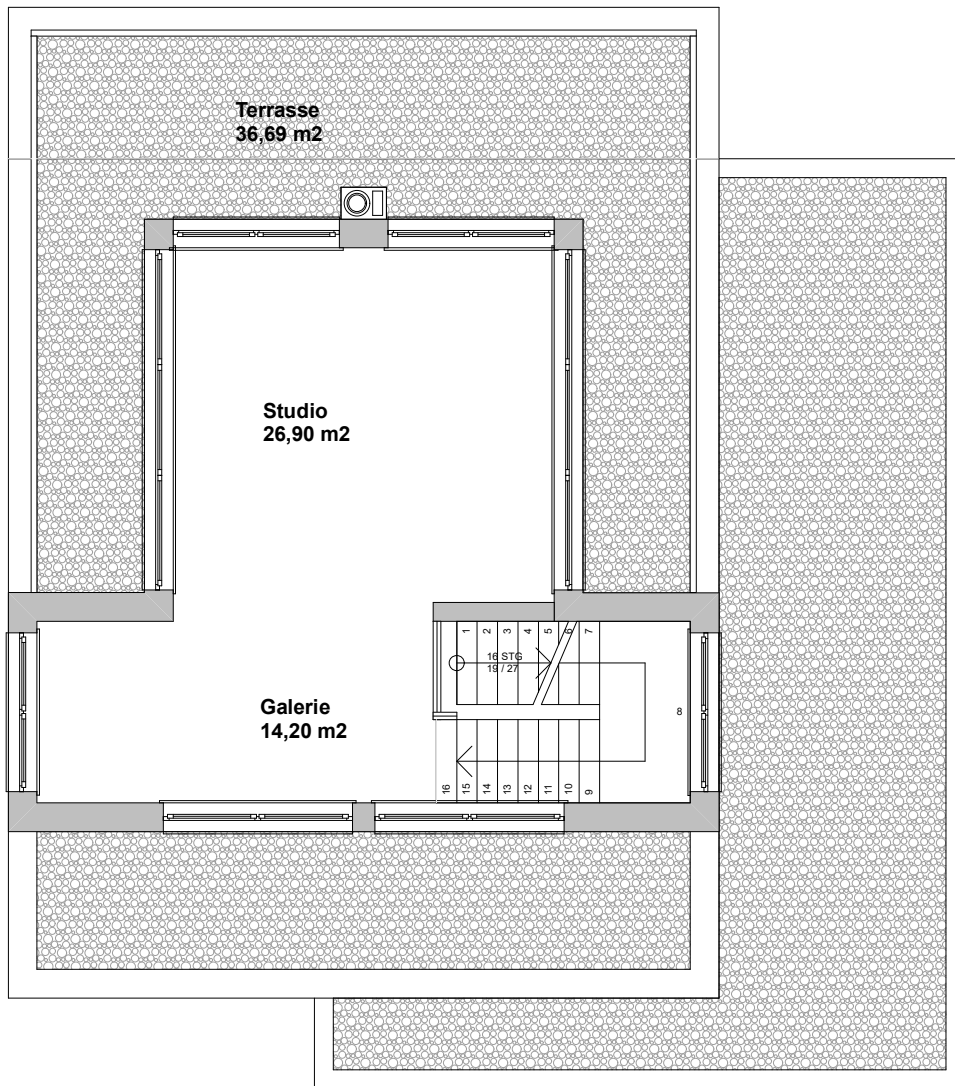
Dachgeschoss M 1:100 - WNF = 41,10 m 2
